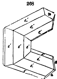
Rutile.
